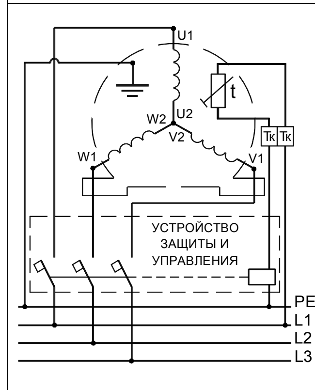
Схема подключения трехфазного электродвигателя вентиляторов
